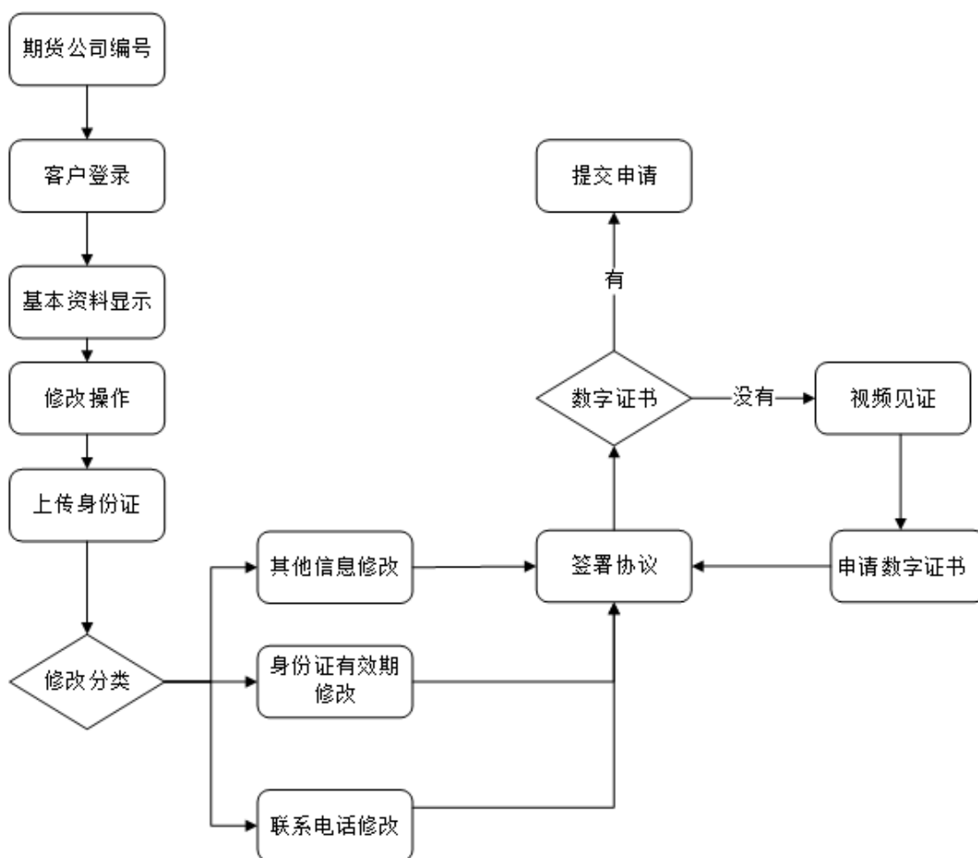
图 1 前端我的基本资料流程
